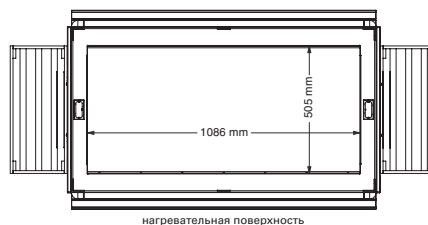
нагревательная поверхность
